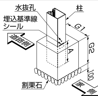
図1-3 独立基礎の場合
