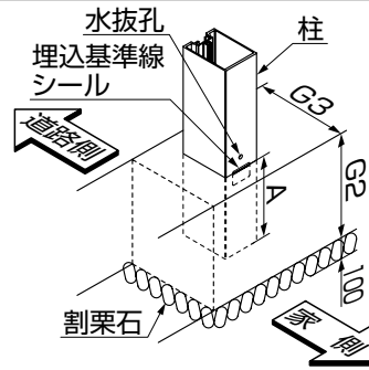
図1-4 連続基礎の場合
